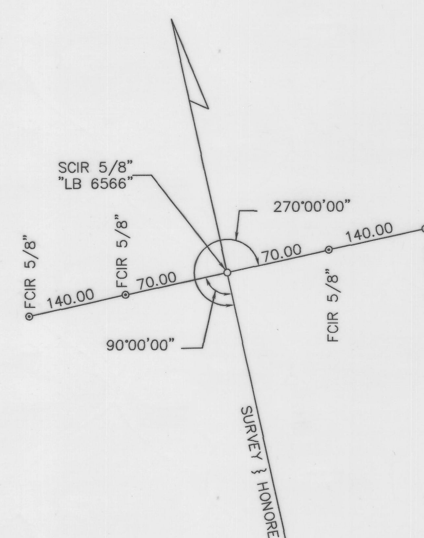
P.O.T. STA. 663+00
