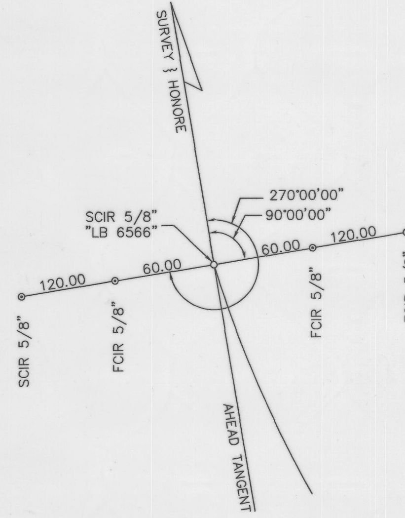
P.T. STA. 651+19.30
