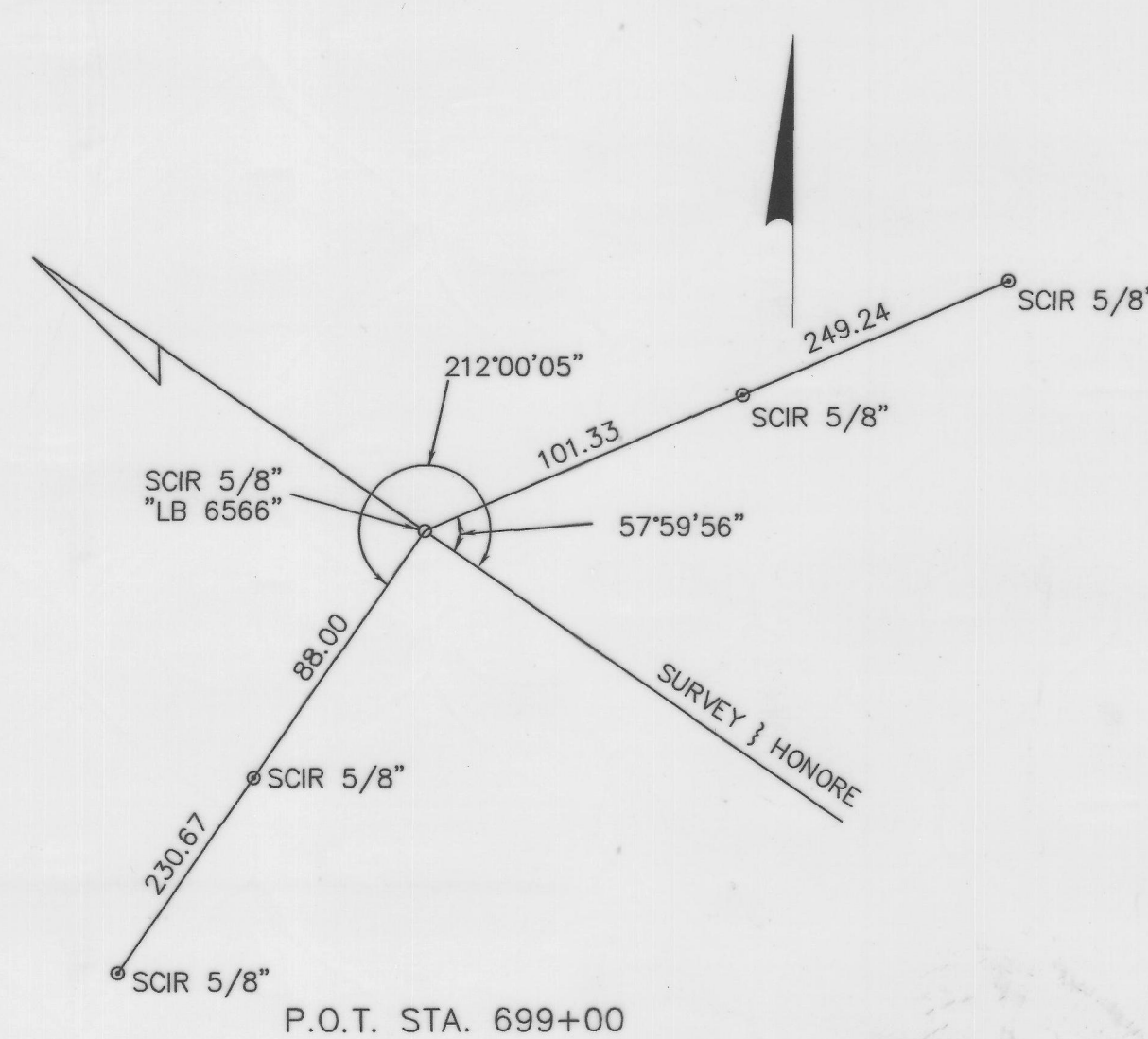
P.O.T. STA. 699+00
