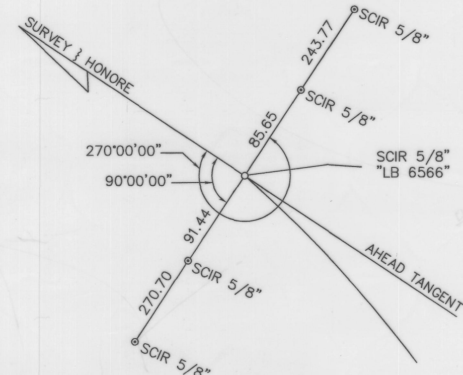
P.T. STA. 690+98.79
