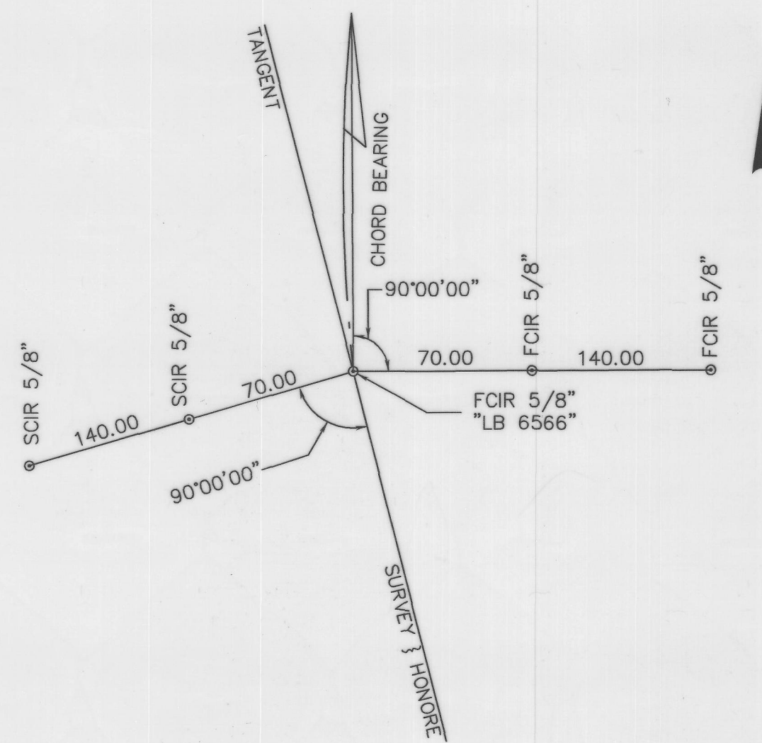
P.C. STA. 640+17.61
