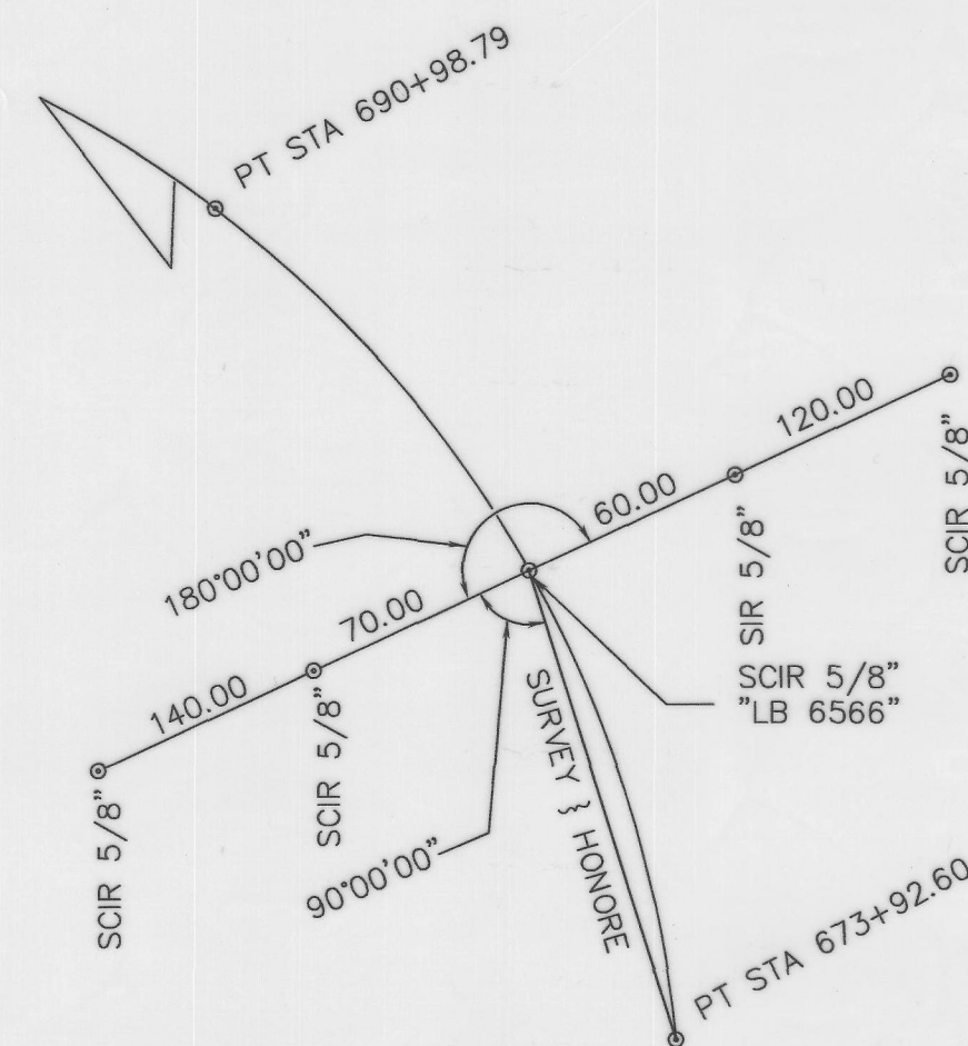
P.O.C. STA. 682+00
