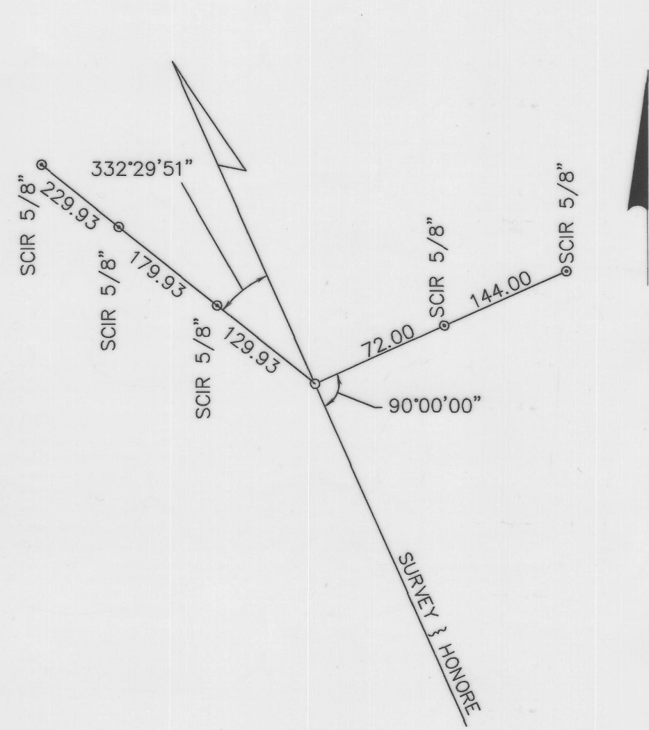
B.O.S. STA. 638+02.37
