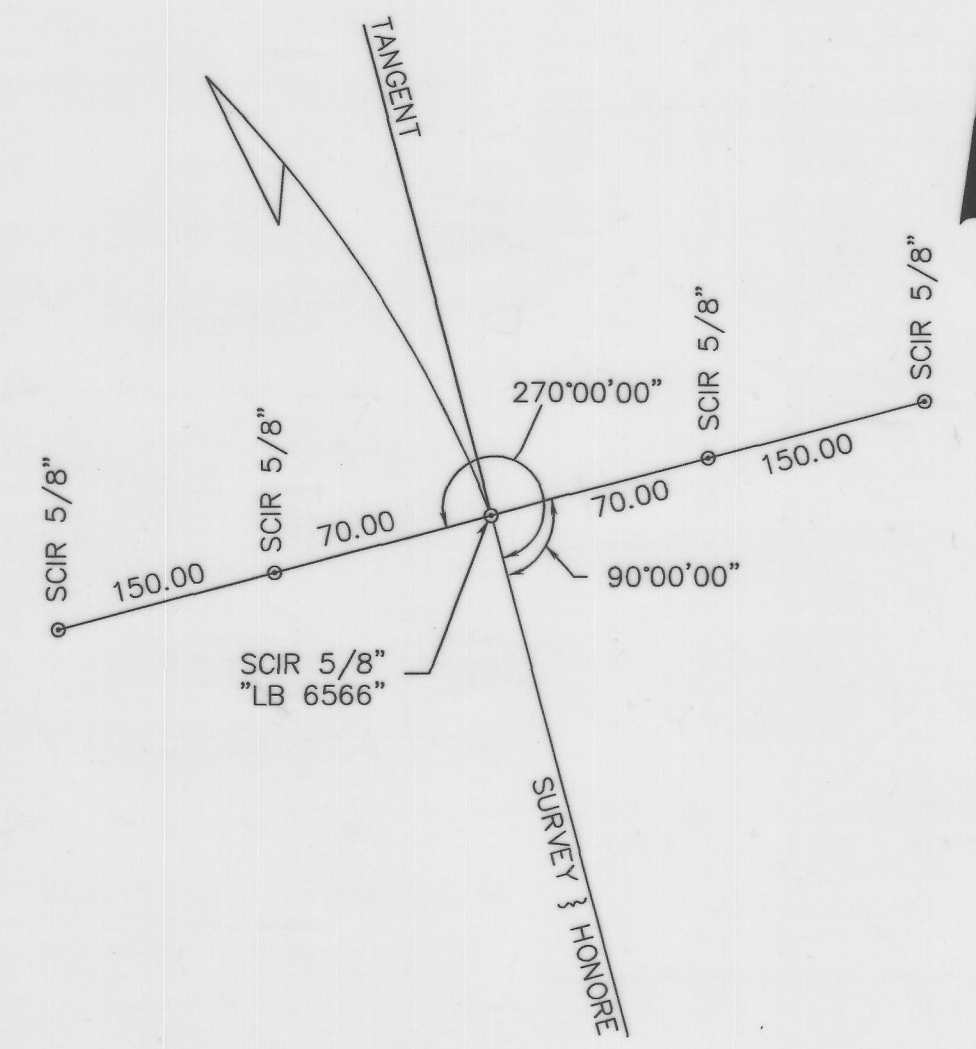
P.C. STA. 673+92.60
